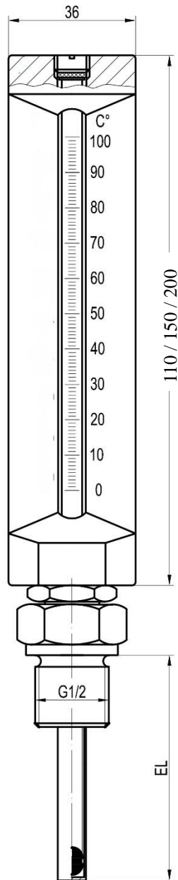
Typ 2985 nach DIN 16185, gerade NG 150 x 36 mm mit Messingschutzrohr zum Einschrauben
