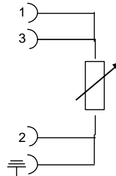
PT-Signal: 4-Leiter
