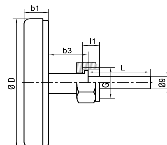
avec écrou-chapeau
