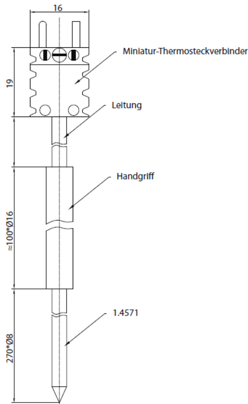
Einstechfühler 2516010-9999
